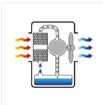
Diagramma di raffreddamento evaporativo Master
